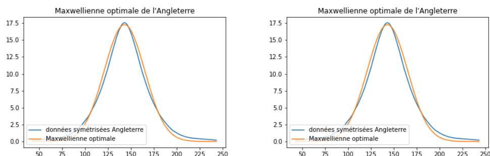
FIGURE 3 – Modèle Maxwellien
